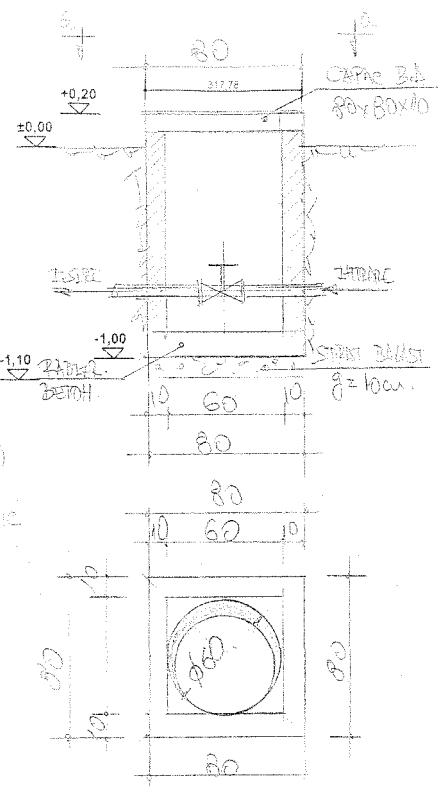
VEDERE A-A
