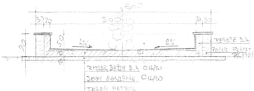
SECTIUNE TRANSVERSALĂ FĂNTÂNĂ ARTEZIANĂ scara 1:50
