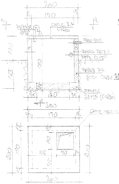
VEDERE A-A
